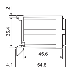
062.07 cu relee
