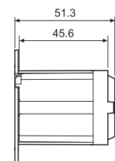
062.05 cu relee
