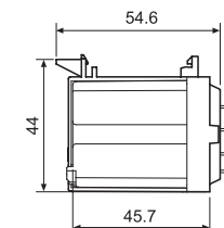
062.08 cu relee
