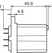
062.10 cu relee
