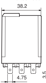
Tipul 62.33 62.33-4300
