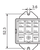
062.05 cu relee
